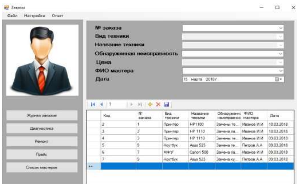
Рисунок 4. Окно диагностики
