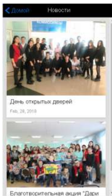
Рисунок 2. Новости
