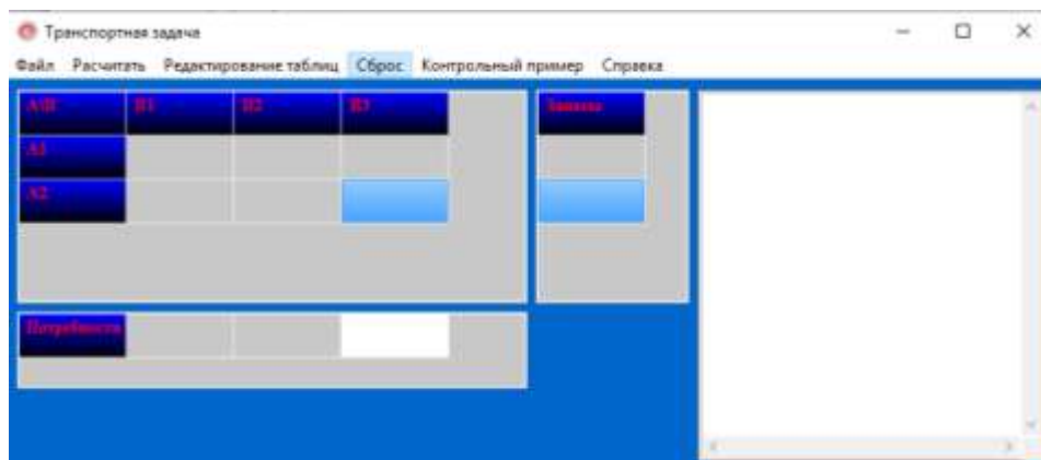
Рисунок 5. Сброс
