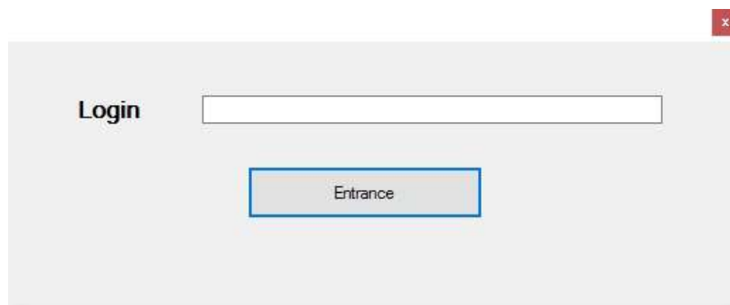
Рисунок 2. Авторизация пользователя
