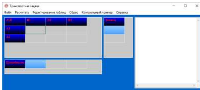
Рисунок 1. Окно приложения
