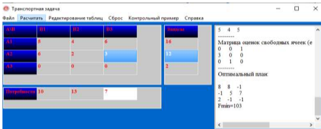
Рисунок 4. Расчет задачи
