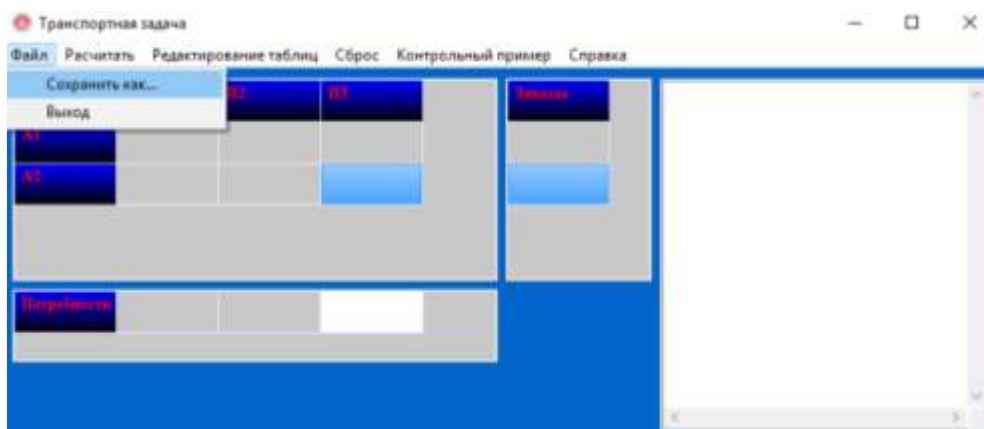
Рисунок 6. Сохранение решения
