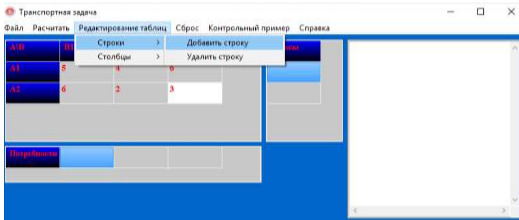
Рисунок 3. Редактирование таблиц
