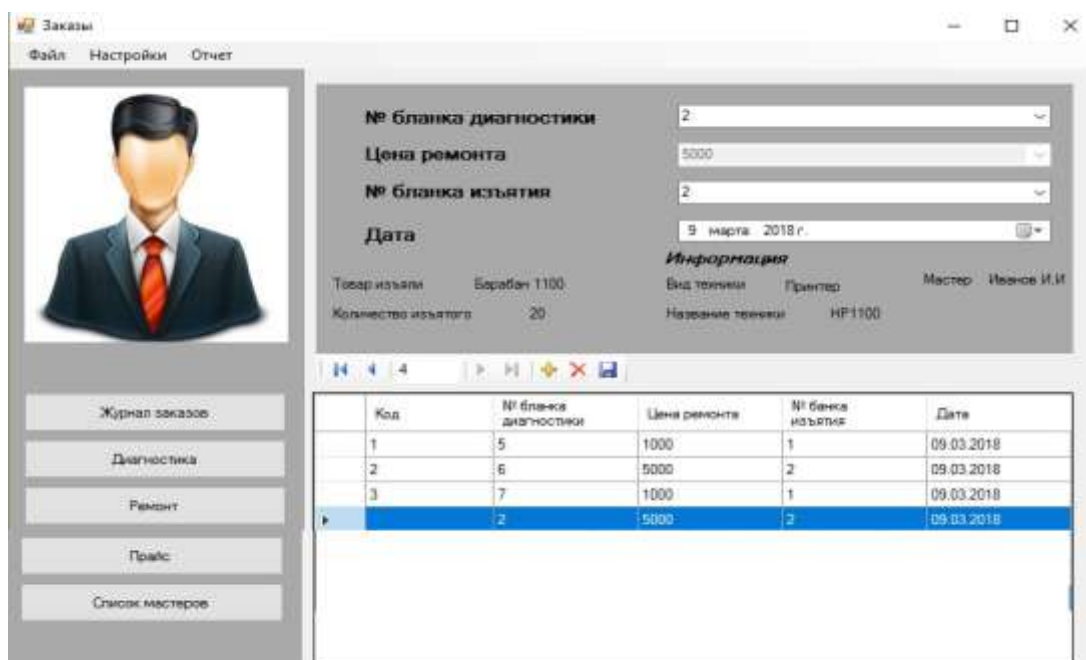
Рисунок 5. Окно «Ремонт»
