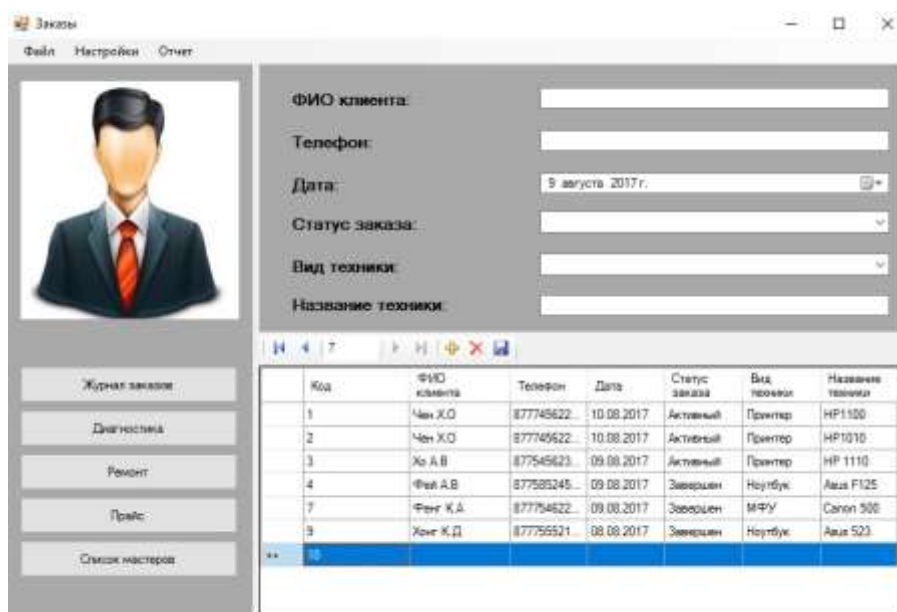
Рисунок 3. Журнал заказов
