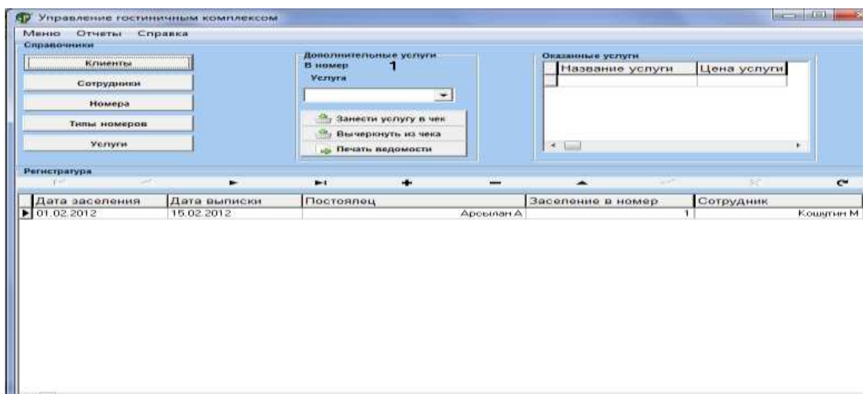
Рисунок 2. Главная форма
