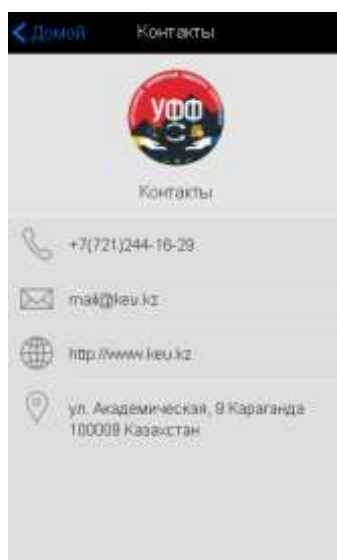
Рисунок 7. Контакты
