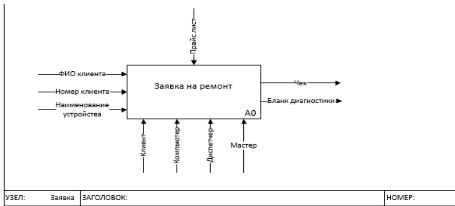
Рисунок 1. Диаграмма IDEF0 «Заявка на ремонт»
